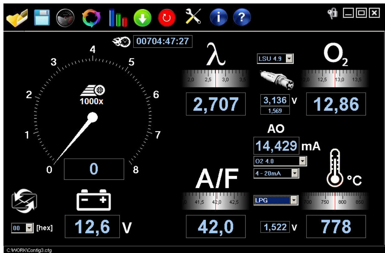
Spuštění vizualizace
